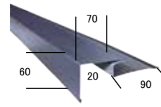
ケラバ捨板
