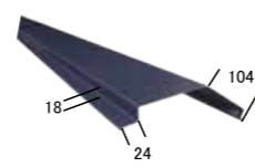
棟カバー
