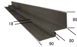
流用壁捨板
