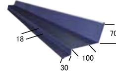
壁際水切り
